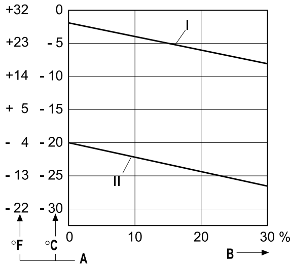
A 1 Zumischung von Petroleum zu Sommerdieselmotorkraftstoff
